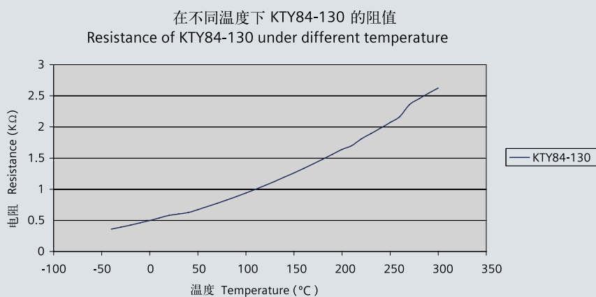
KTY 84-130 温度传感器的特性曲线 KTY84-130 sensor characteristics curve
