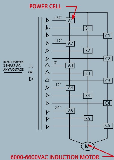
6000-6600VAC INDUCTION MOTOR 6000-6600V 变频器拓扑
