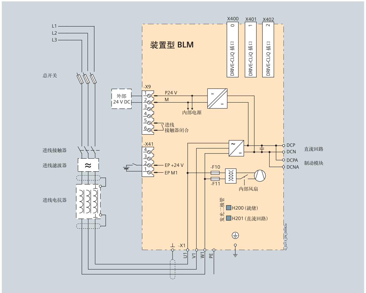
连接示例：装置型基本电源模块
