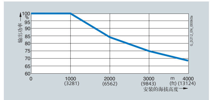
输出功率与安装海拔高度的关系
