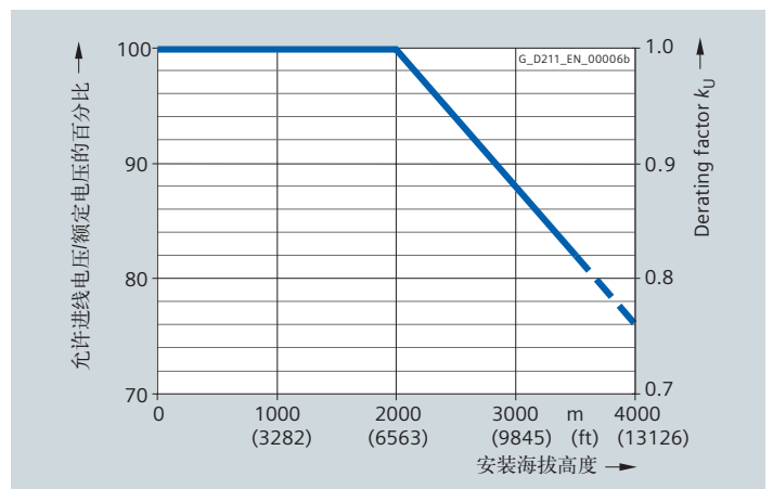
电压降容与安装海拔高度的曲线
