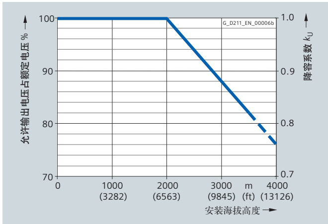
电压降容与安装海拔高度的曲线
